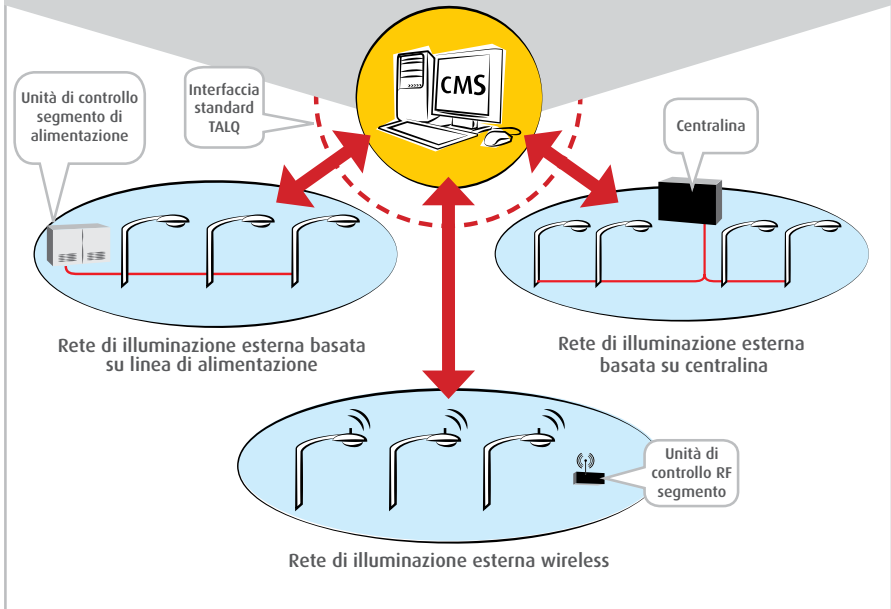
Figura 2 - Architettura di sistema TALQ
